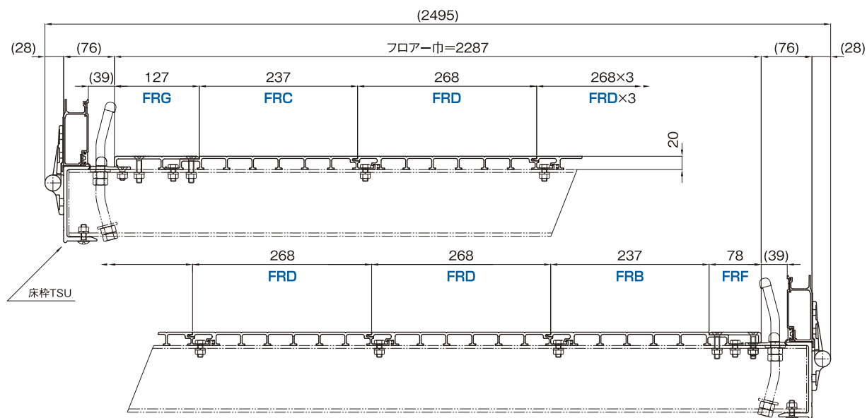
フロア構成例とフロア巾&長さ当り重量
